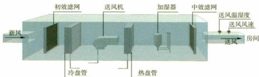
新风空调系统送风示意图
