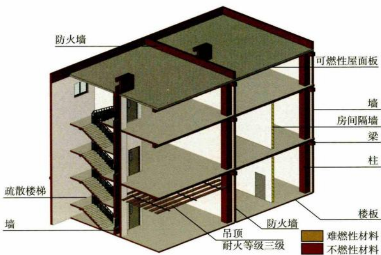
5.1.1 图示 3：耐火等级三级
