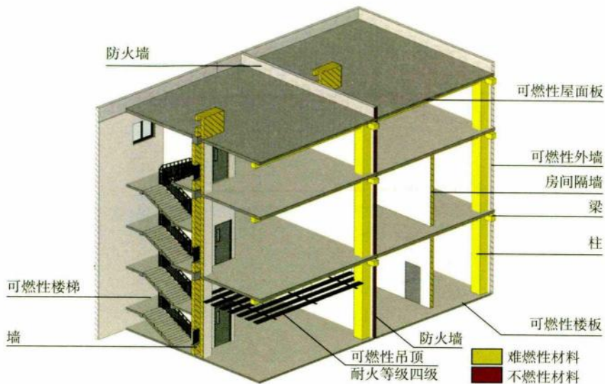
5.1.1 图示 4：耐火等级四级
