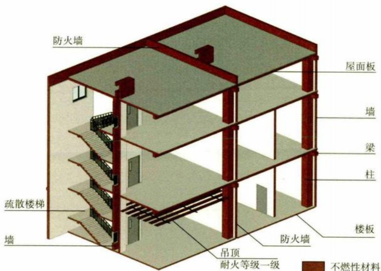
5.1.1 图示 1: 耐火等级一级
