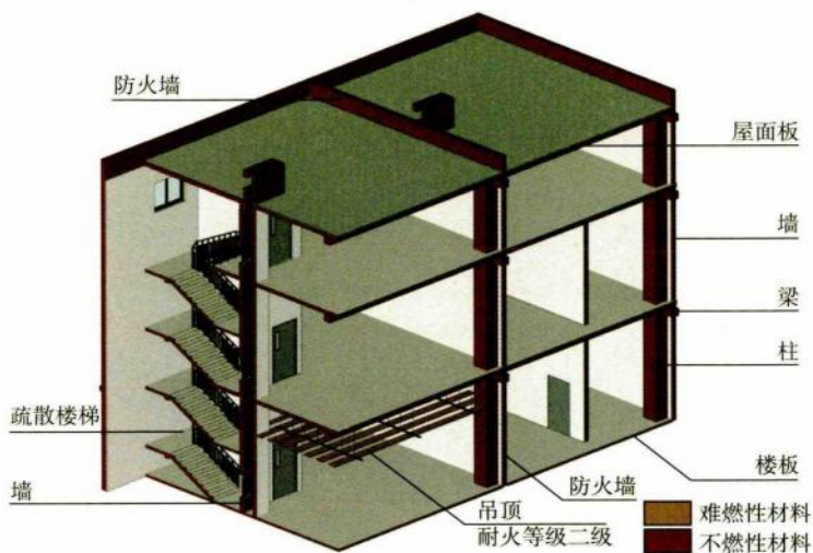
5.1.1 图示 2：耐火等级二级
