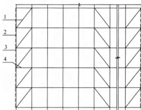
图 6.3.5 斜杆搭设示意
