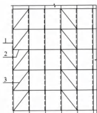
(a) 立面图
