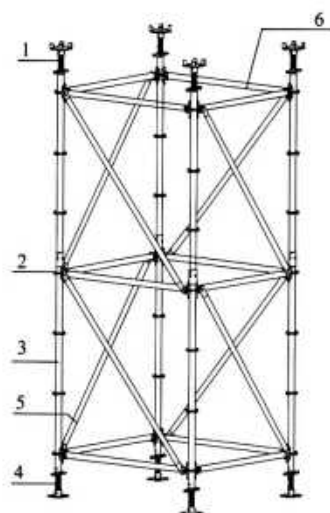
图 3 承插型盘扣式钢管脚手架示意三
