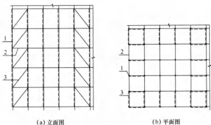
图 6.2.2-4 间隔 3 跨形式支撑架斜杆设置
