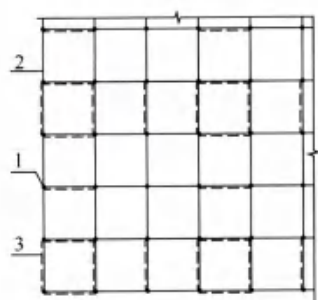
(b) 平面图
