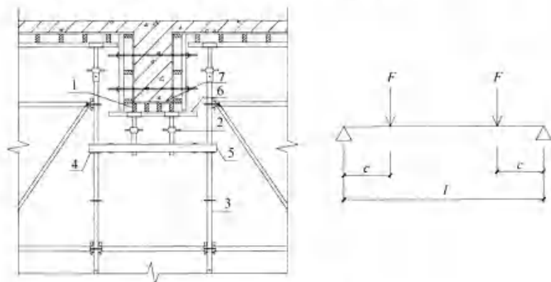
图4 双槽托梁承载力计算示意
