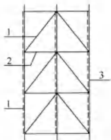
图 5.1.4 独立方塔架
