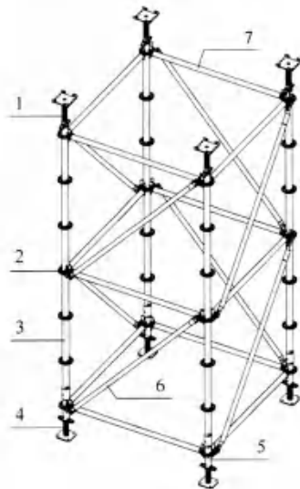
图 2 承插型盘扣式钢管 脚手架示意二
