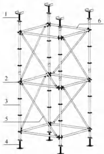
图 1 承插型盘扣式钢管 脚手架示意一
