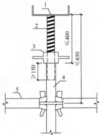
图 6.2.4 可调托撑伸出顶层水平杆的悬臂长度
