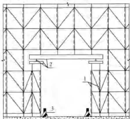
图 6.2.9 支撑架人行通道设置
