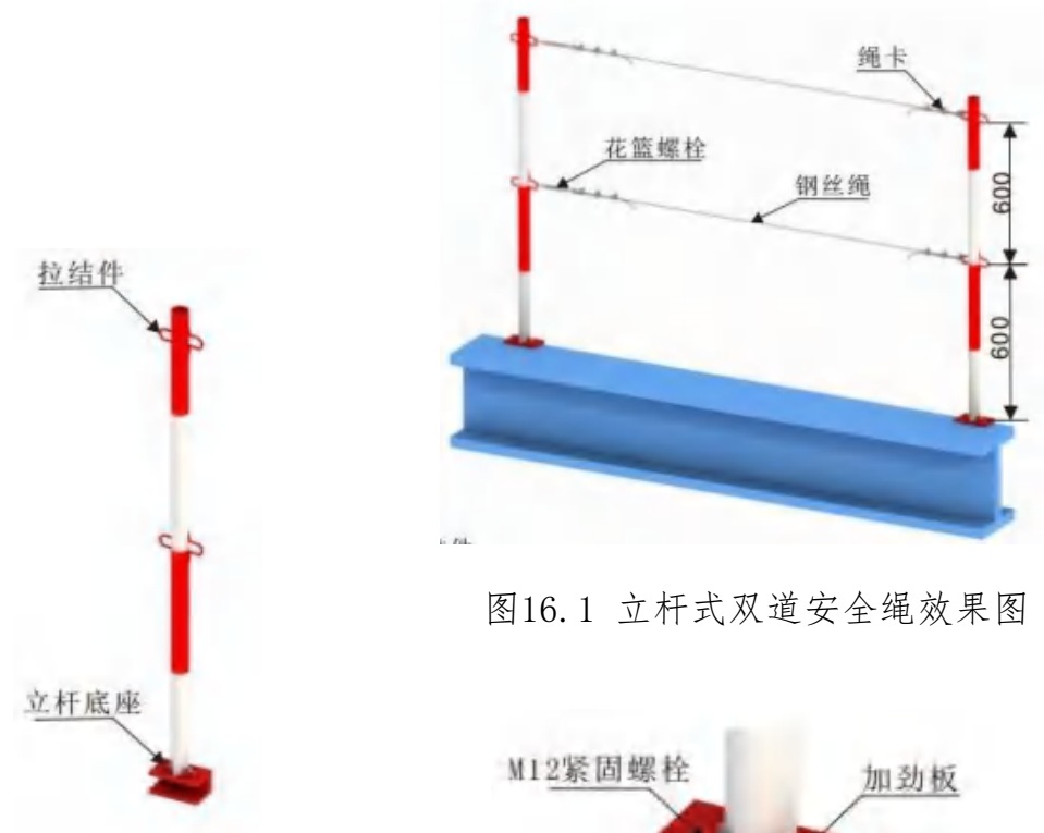
图16.3 立杆效果图
