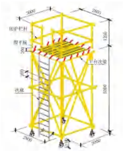
图2.1 操作平台示意图（一）
