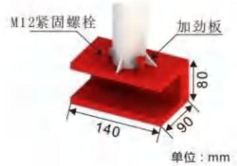
图16.2 立杆及底部夹具
