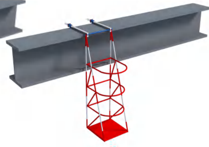
图4.4 焊接吊笼效果图
