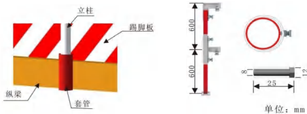
图12.2 立柱底座连接点
