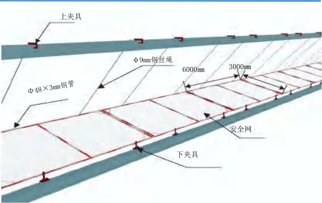
图8.1 外挑网效果图
