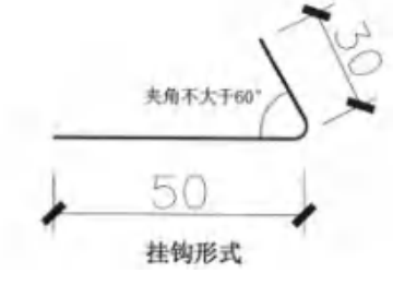
图5.2 弯钩详图
