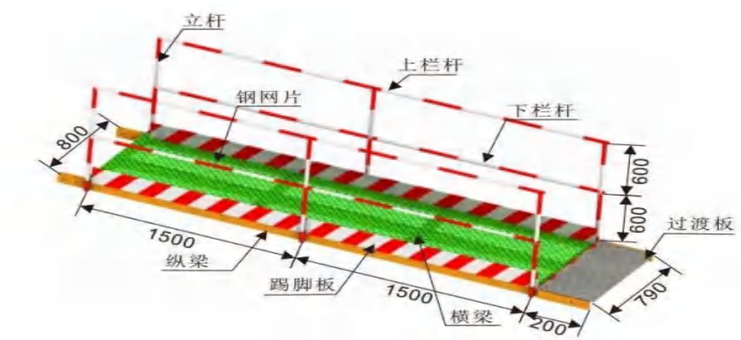
图12.1 钢制组装通道效果图
