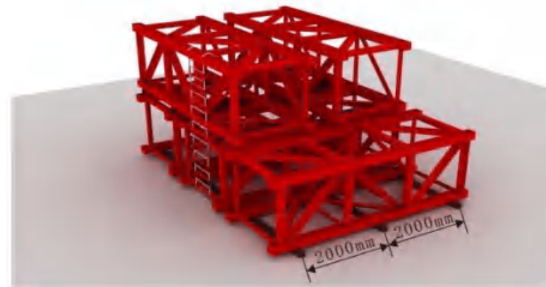
图5.2 胎架卧放示意图
