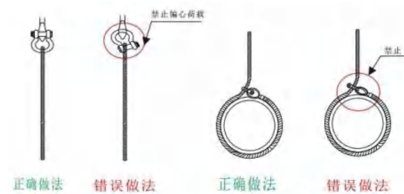
图5.3 卸扣偏心荷载示意图
