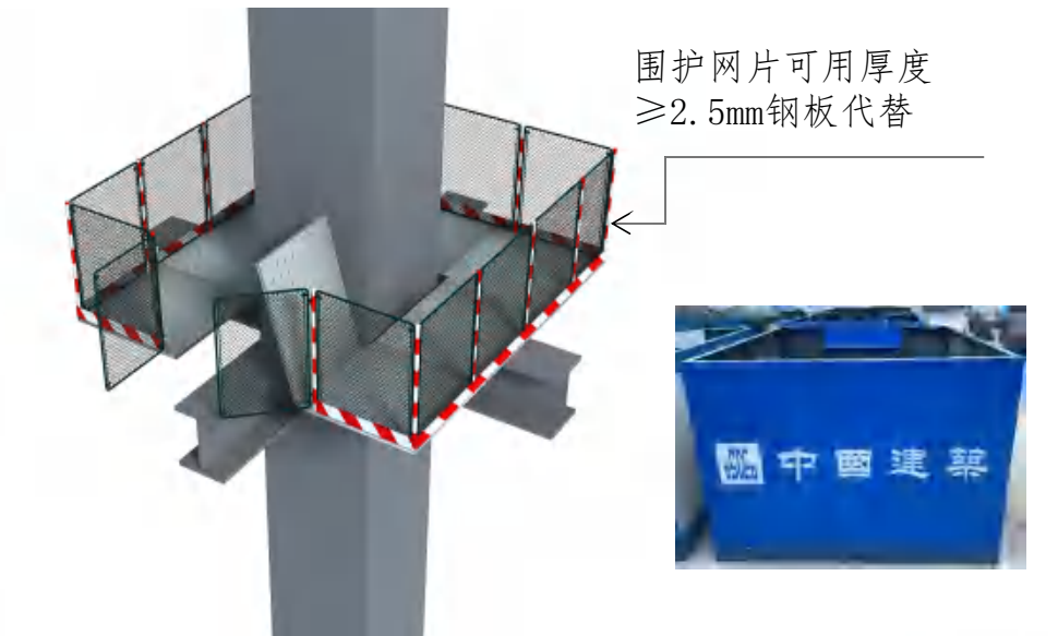
图1.1 操作平台示意图
