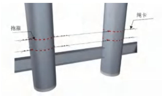
图14.1 双道安全绳-圆形柱示意图
