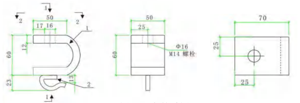
图5.4 夹具详图
