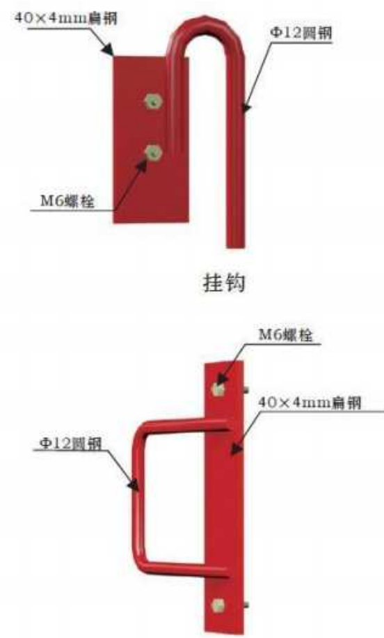
图9.2 局部示意图
