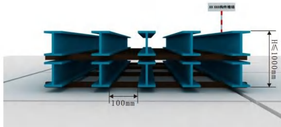
图3.2 侧面示意图
