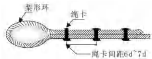
图14.3 绳卡布置详图
