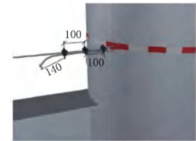
图14.2 绳卡布置示意图
