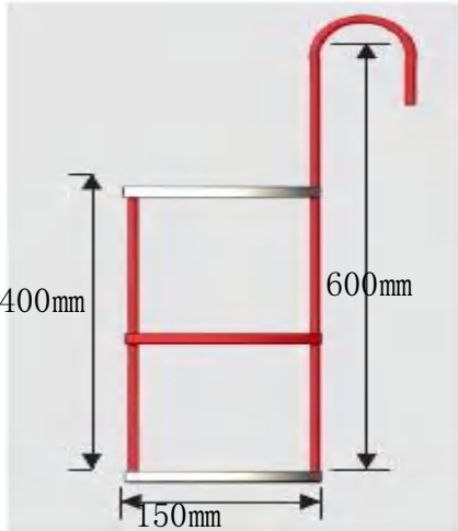
图2.3 挂笼侧视图
